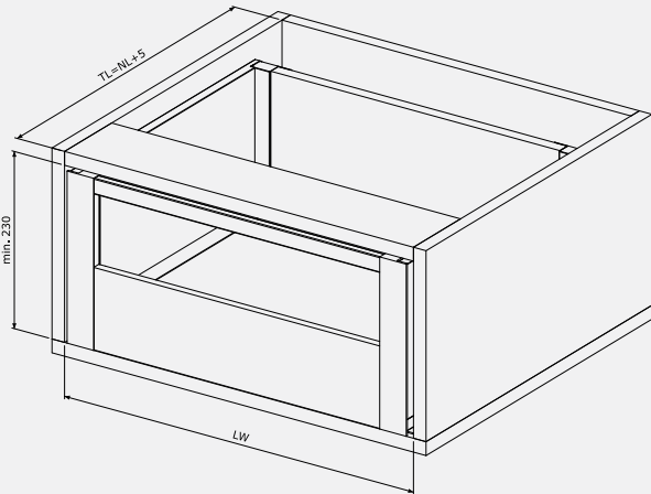
Загальні розміри
