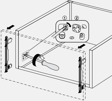
Висота царги 199 мм (два кроки)
