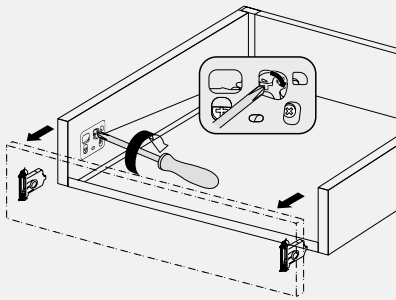
Висота царги 84 та 135 мм (один крок)
