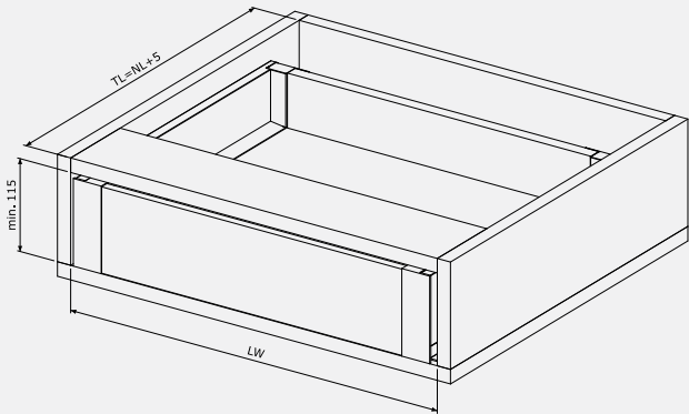
Загальні розміри
